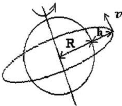
1-расм. Йўлдошнинг Ер сиртидан h баландликдаги ҳаракати
