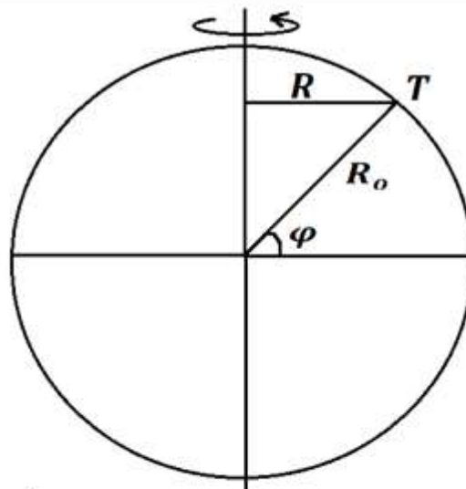
2.1-расм. Тошкент турган нуқтанинг Ер билан биргаликда айланиши
